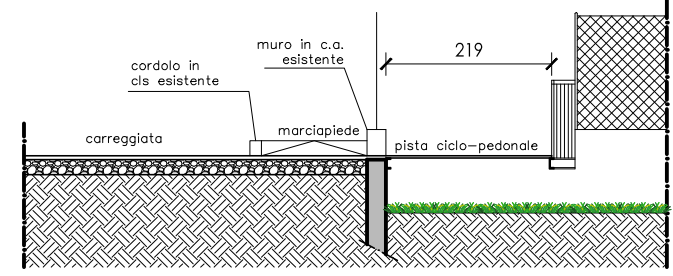
Stato di Progetto SEZ. 7 prog. 218.0 m
