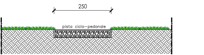
Stato di Progetto SEZ. 8 prog. 262.0 m
