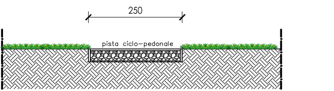
Stato di Progetto SEZ. 7 prog. 218.0 m
